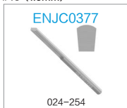
美国GRS GlenSteel® 锥形平雕刻刀 GRS® GlenSteel® Tapered Flat #43 (1.6mm)
